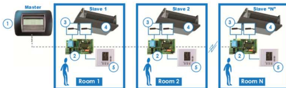
Master-Slave per la Regolazione di Zona con parametri ritrabili Master-Slave for the Regulation of Area with recalibrated parameters
