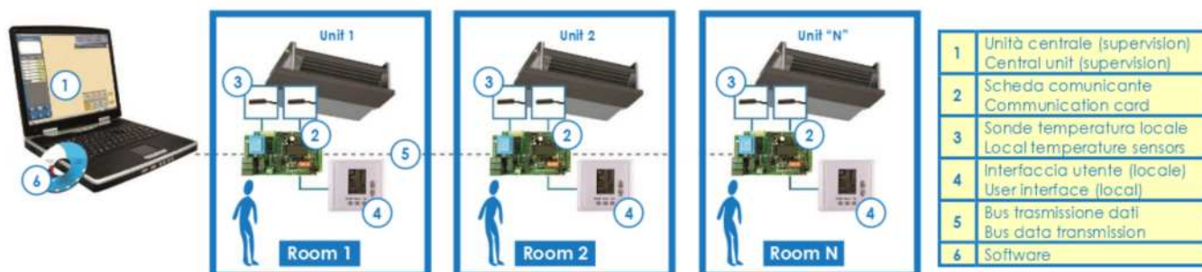
Regolazione con Comunicazione (BMS) Regulation with Communication (BMS)
