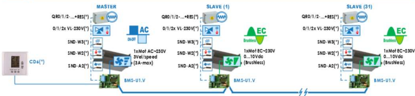
Fig.6 MASTER-SLAVE (Regolazione di Zona con SET-POINT fisso), (Regulation of the Area with fixed SET-POINT)
